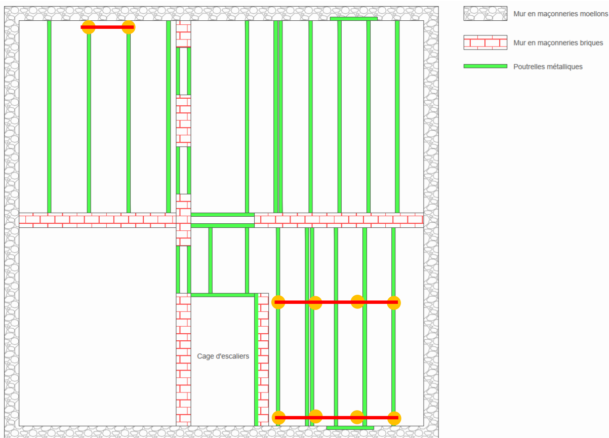
Plan de principe d'étaielement
