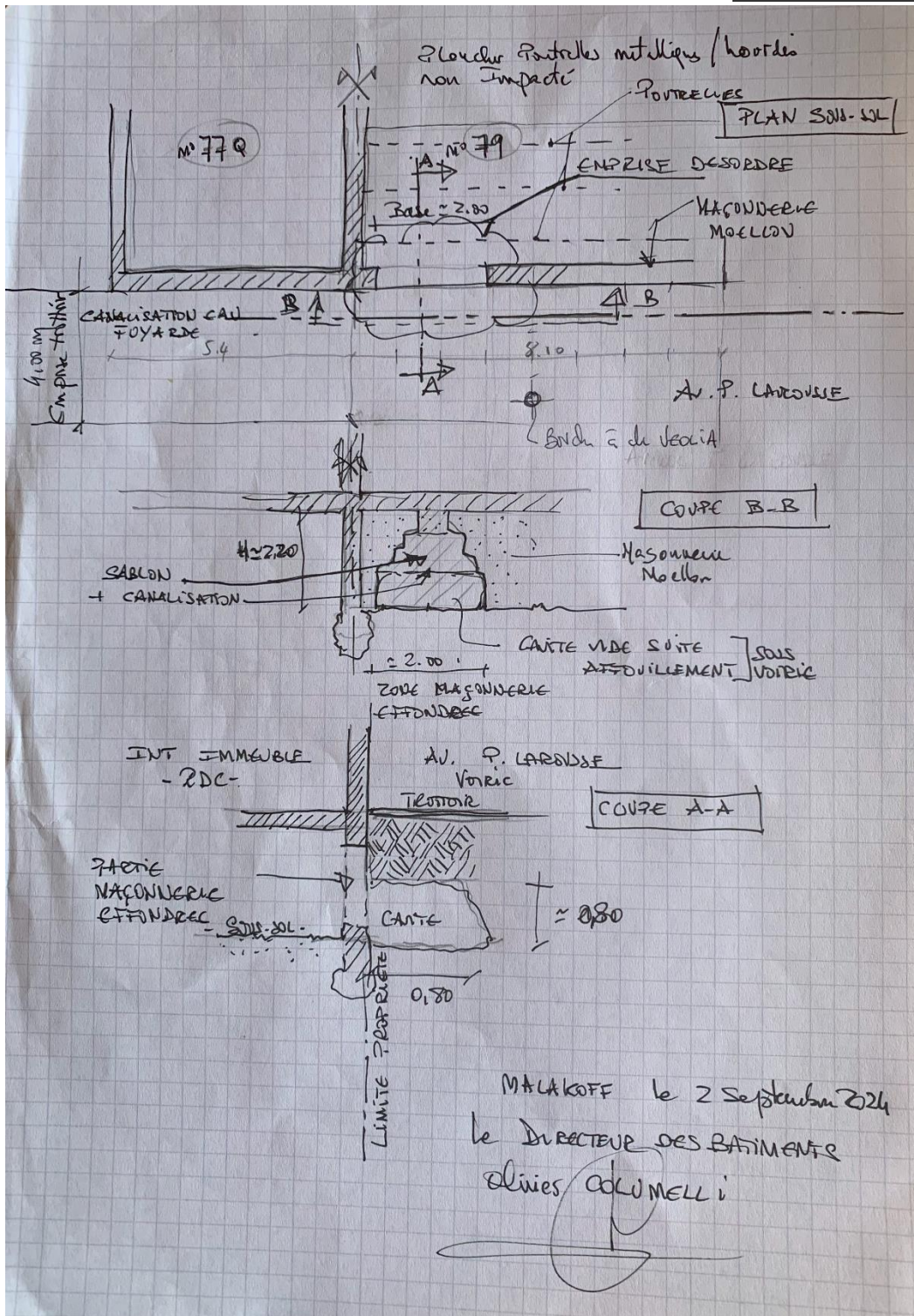
PLAN SCHEMATIQUE
