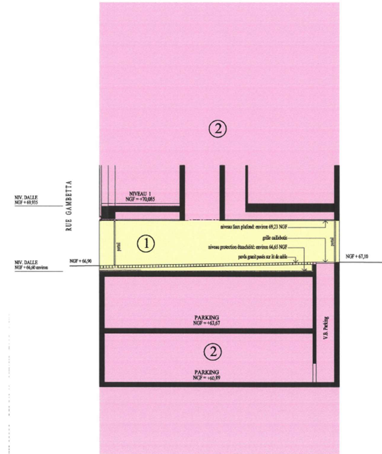
Plan en coupe
