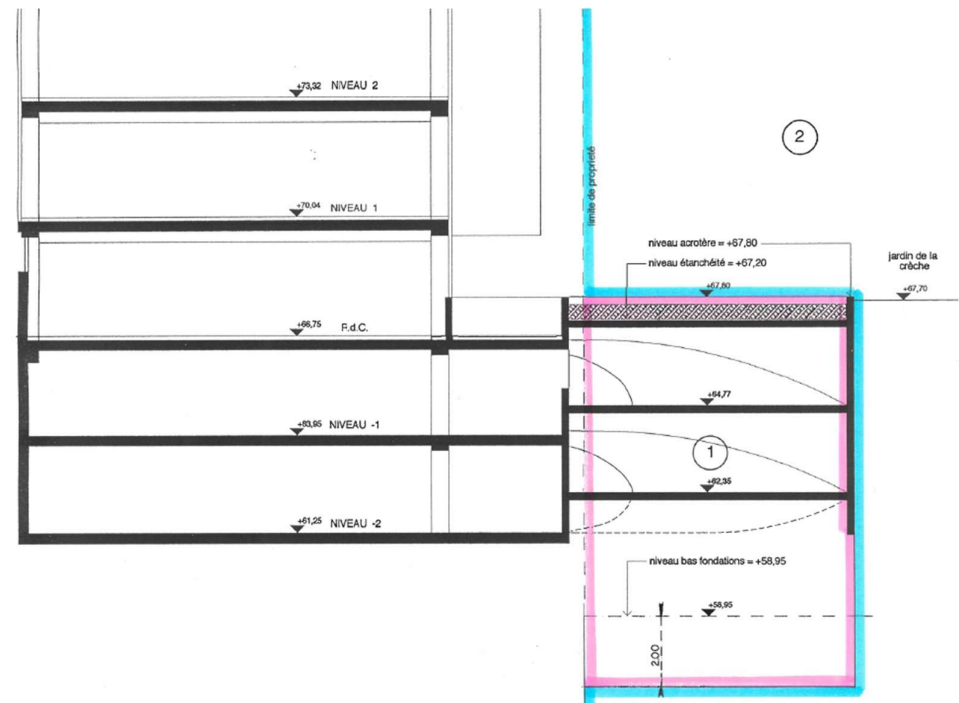
Plan en coupe
